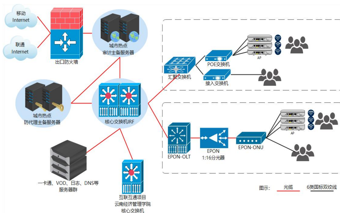
图 33 校园网拓扑结构
