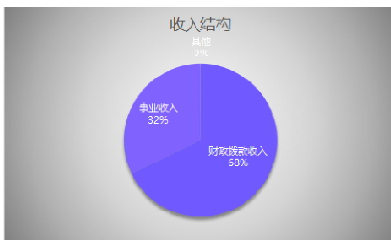
图 6—2 收入结构图
