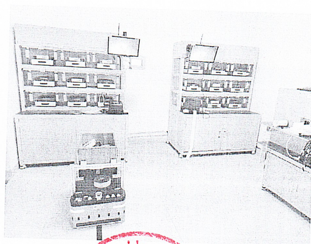
图 7 智能货架和 AGV 小车
